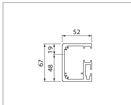
TP710/1 Guía / montaje a muro
