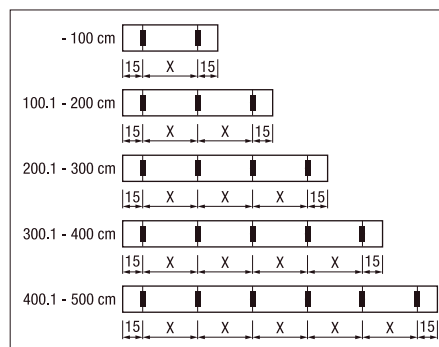
Configuración y número de abrazaderas de fijación / punzones o clips
