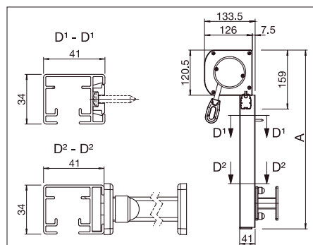
VS5200/1: Instalación a pared con clips A = Altura total
