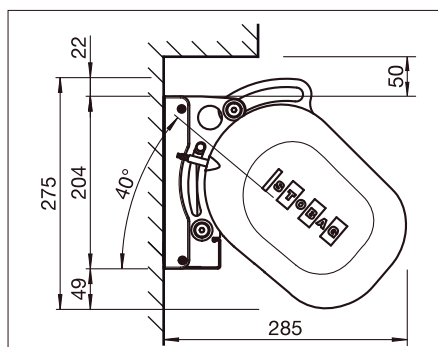
Instalación a pared 40°
