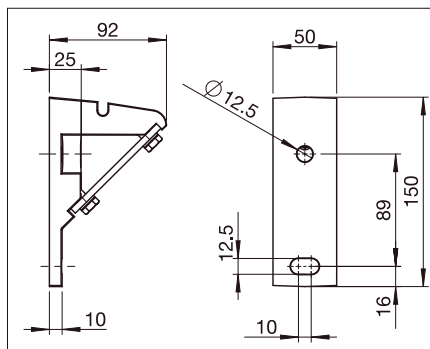
S831/5 Soportes para viga (desde el frente)
