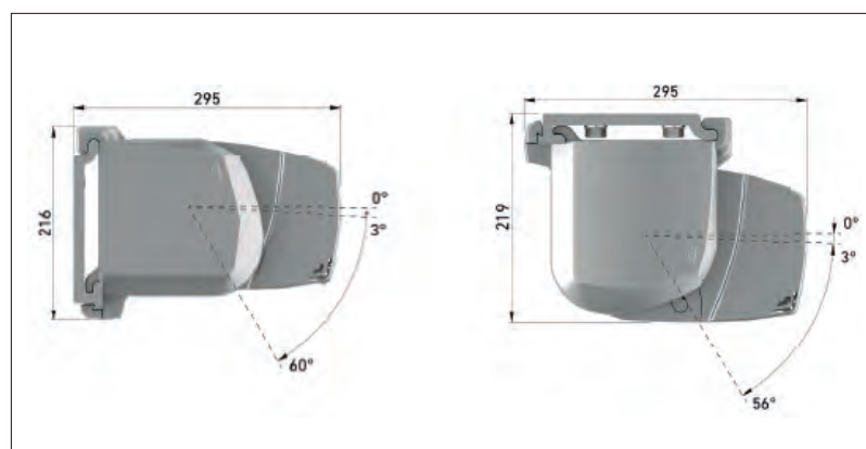
fijación a muro
