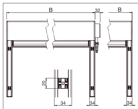
Disposición de los soportes con sistema de clips B = Total width
