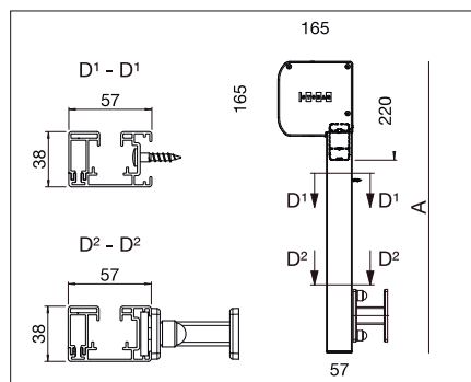
VS5600 / 1: Montaje en pared mediante roscado directo y con soportes de montaje - A = Altura total
