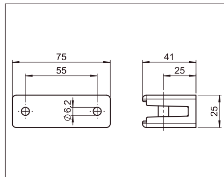
SR416 Pestillo
