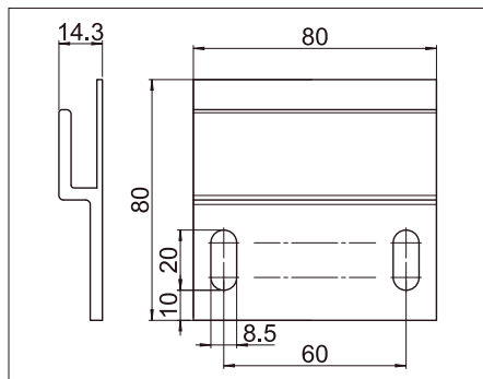
SR606 Instalación a pared
