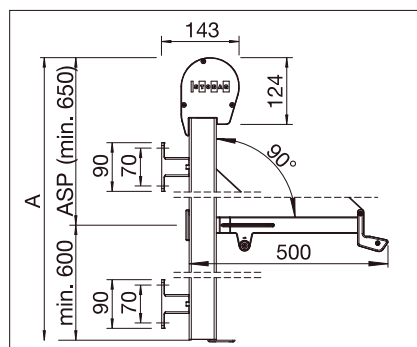
Al aire con cofre redondo
