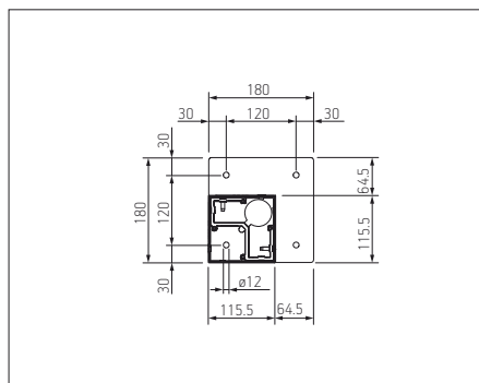
Placa base (modelo de ángulo)
