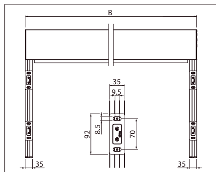
Disposición de los soportes con sistema de clips B = Ancho total
