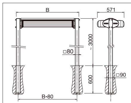
Tacos al suelo
