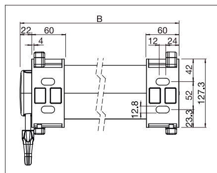
Plano de montaje con cambio de engranajes Soporte S721/1
