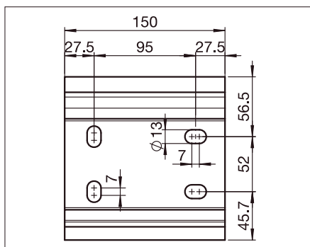
S721/2 Perfil de soporte L= 150
