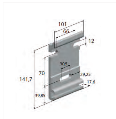
detalle soportes a muro
