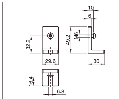
S307 Soporte de fijación
