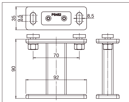
PS452/1 Soporte
