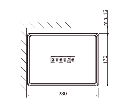
Montaje a muro
