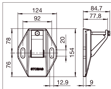
S821/1 Soportes techo/muro
