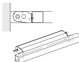
2 motor interior sobre perfil portante
