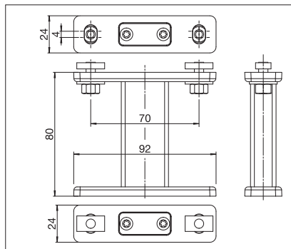
FS601/3 Soporte de fijación
