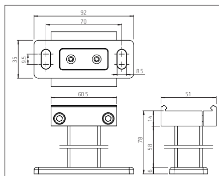
PS826-1 Soporte de fijación estándar (cajón pequeño)
