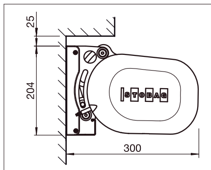
instalación a pared
