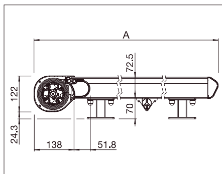
Instalación sobre sub estructura A = Proyección
