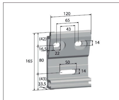
fijación a muro para taco químico
