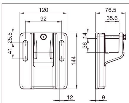
S221/1 Soporte para techo
