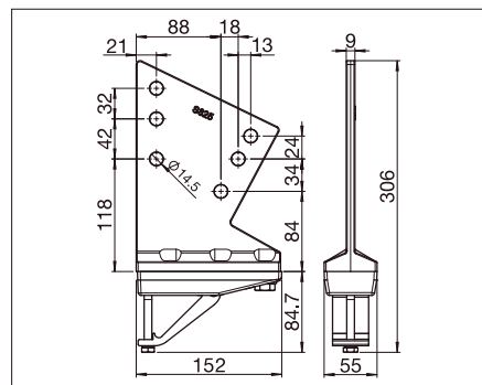
S825 Soportes pequeños techo/muro
