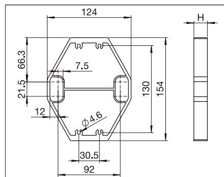
S821/1.. Distancia placas
