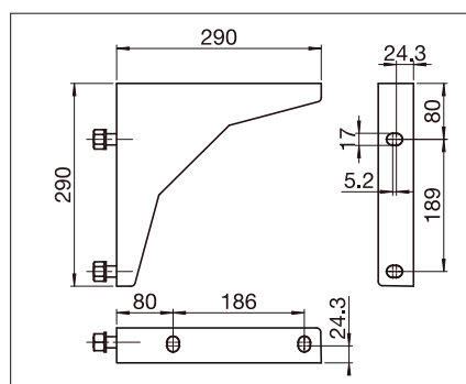
S346 Soporte para techo
