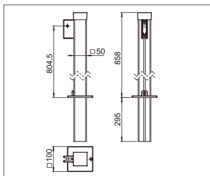
SR414/2 Kit poste para empotrar
