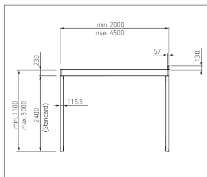
Vista frontal de 1 módulo con tejido de lamas modulares
