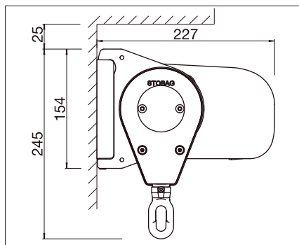
Instalación a pared Rail frontal redondeado
