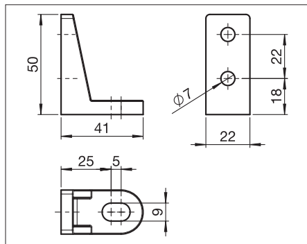
US120-2 Soporte de fijación a muro
