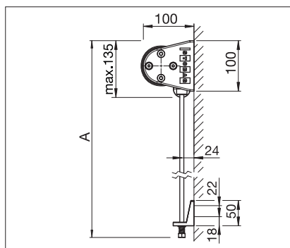
S4110/2 Montaje a muro
