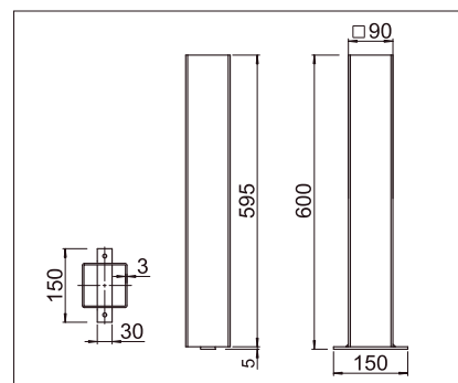
OS615 Tacos para suelo
