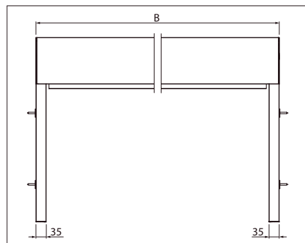
Disposición de los soportes, con motor B = Ancho total
