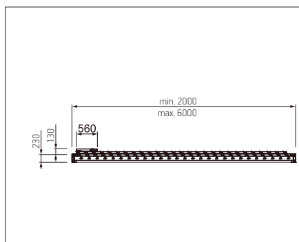
Vista lateral TR4520
