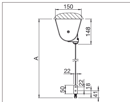
US3910/1 Instalación superior
