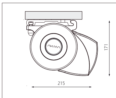
fijación a techo
