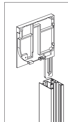
Detalle espiga tapa lateral y guía de 2 cuerpos
