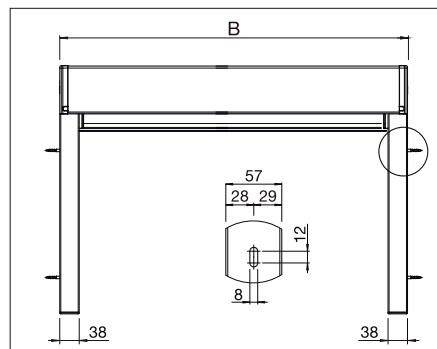
Dibujo de la instalación: al techo mediante montaje directo B = Anchura total
