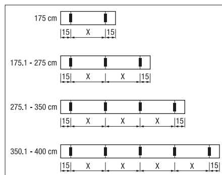
Distribución y número de soportes / agujeros
