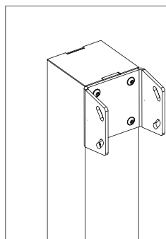
soporte exterior para guía y perfil 120x120
