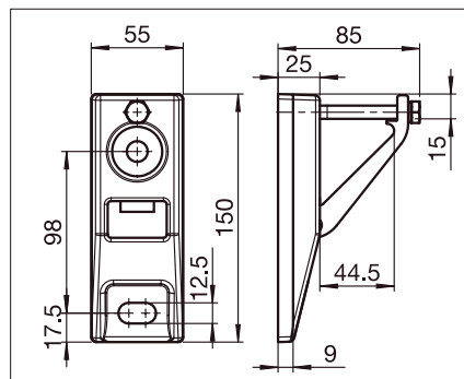
S821/2 Muro/ Soporte pequeño para techo
