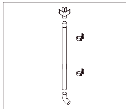
Canaleta para el agua
