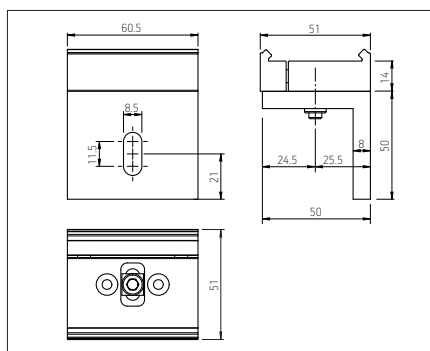
PS815 Soporte de fijación para techo
