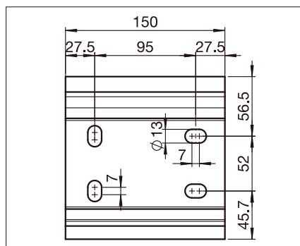
S721/2 Soporte
