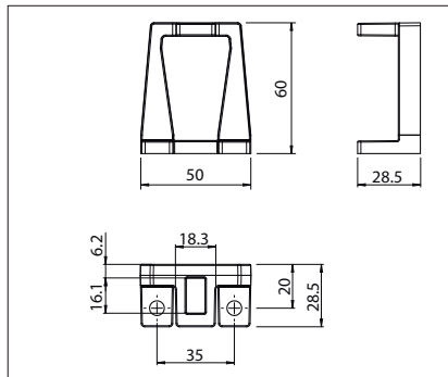
US120-1 Soporte
