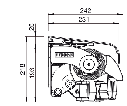
Instalación a pared con tejadillo (SG217 front rail)
