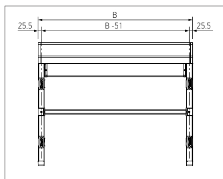
Plano de montaje B = largo total
