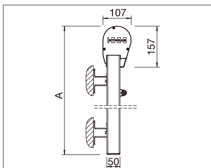
Retraído con cofre redondo
