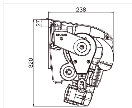
S8133 Instalación a pared con tejadillo
