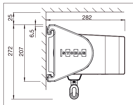
Vista lateral instalación a pared - cuadrado
