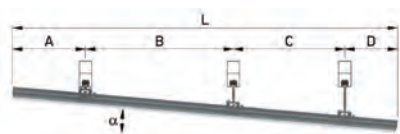
sistema entre paredes
