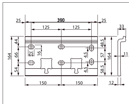
Soporte largo para vigas
