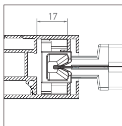
Sección guía ZIP
