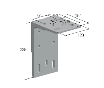
detalle soportes a techo (no incluido)
