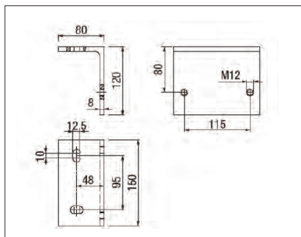
P333 Soporte para fijación a techo
