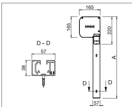
VS5600/2: Instalación a pared A = Altura total
