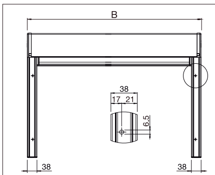
Plano de montaje: montaje a pared directo por tornillo B = Anchura total
