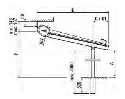
Montaje a muro con placa base
