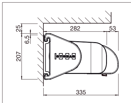
Fijación a pared con cenefa de caída Rail frontal redondeado
