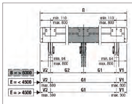
Plano de montaje | B= largo total
