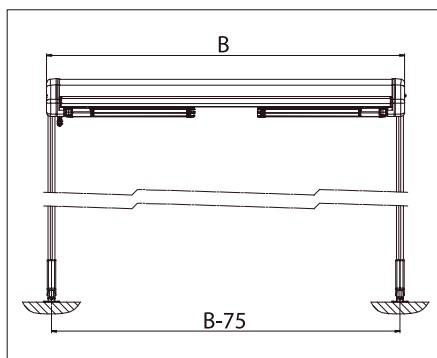
Version OS416/1 base de ángulo recto
