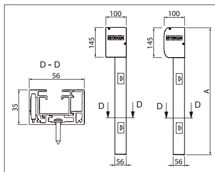
Montaje entre paredes A = Altura total
