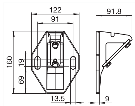
S831/3 Muro/ Soportes para techo(vista frontal)
