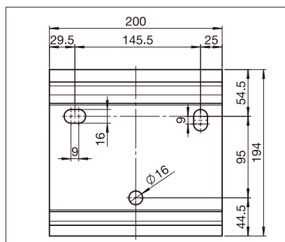
S563/1 Perfil de soporte L = 200
