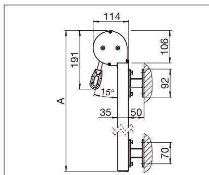
US3910/3 Montaje incorporado
