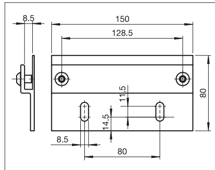
US206 Placa de instalación
