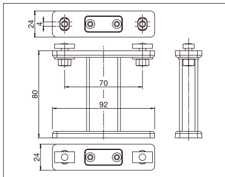
FS601/3 Soporte de fijación
