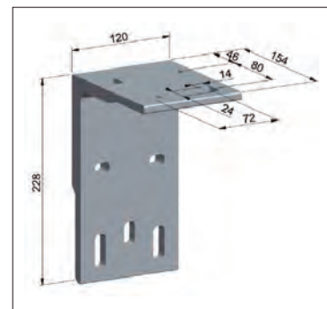
fijación a techo (+ placa frontal)
