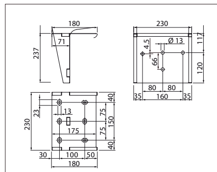
Herraje para montaje a techo
