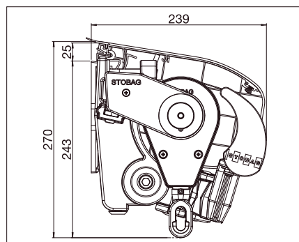
S8130 Instalación a pared con tejadillo S877/2
