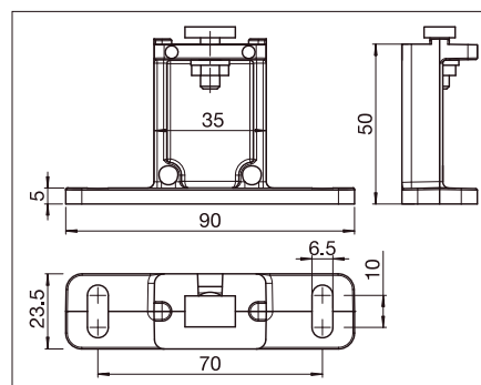
FS602/1 Soporte
