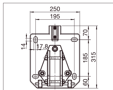
S340 Pie de la base S341 Soportes intermedios de pared / techo
