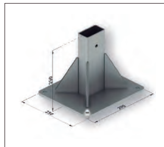
Base soporte
