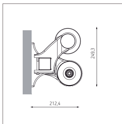
fijación a muro
