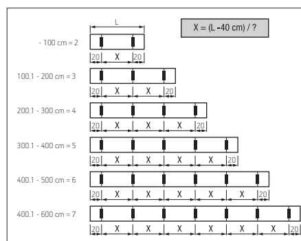
Reparto y nº de soportes con ZIP
