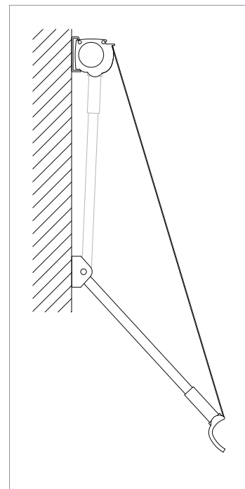
con brazo de 140, apertura máxima de 140°
