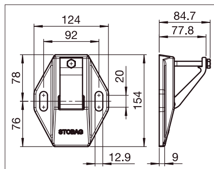
S821/1 Muro/Soporne instalación a techo
