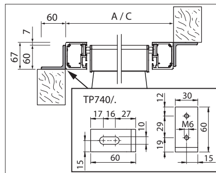
Esquema de montaje bajo techo o en fachada
