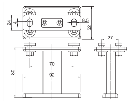
FS601/4 Soporte de fijación doble
