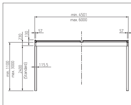
Vista frontal de 2 módulos con tejido de lamas modulares
