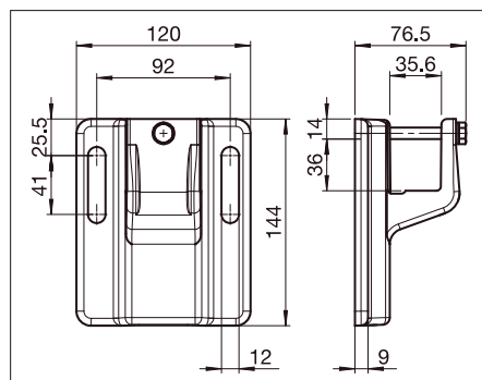
S221/1 Soporte
