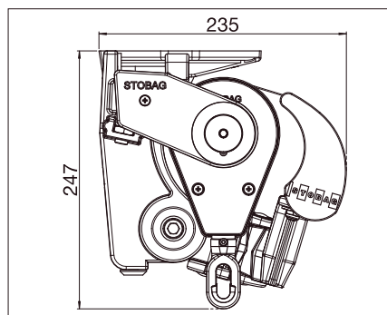
S8130 Instalación a techo
