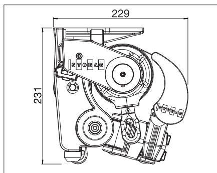
S8135 Instalación entre muros
