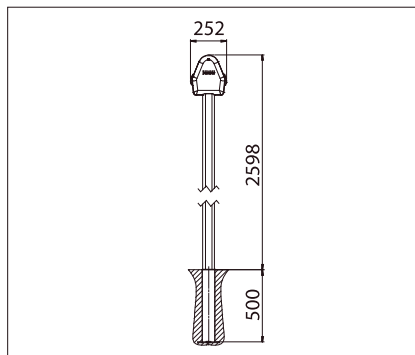
Version de 2 postes OS416/2 con camisa OS315
