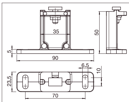
FS602/1 Soporte de fijación
