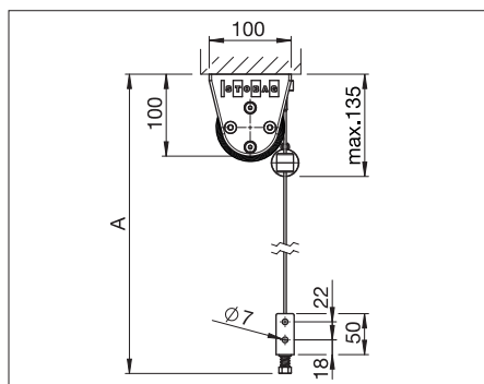
S4110/1 Montaje a techo
