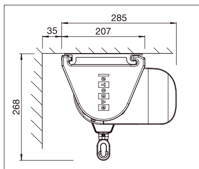
Vista lateral instalación a techo - redondeado
