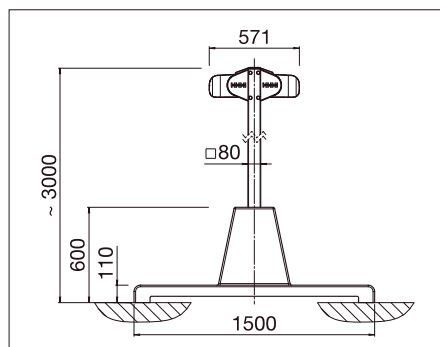
Con zócalos de hormigón
