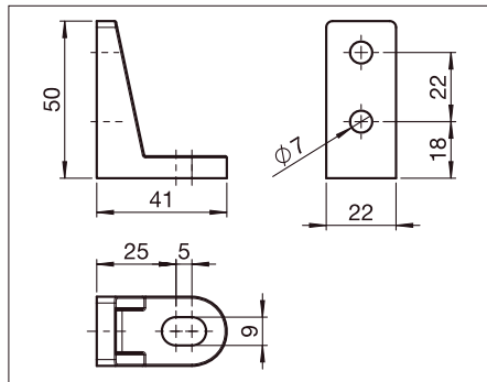
US120-2 Soporte
