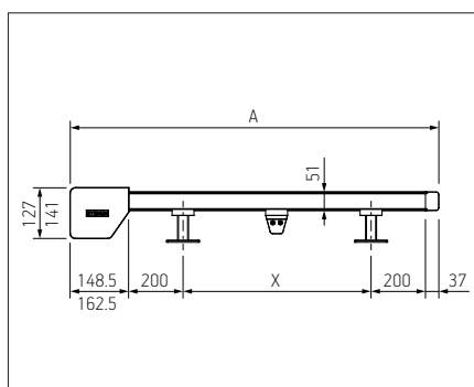
Vista lateral A = salida
