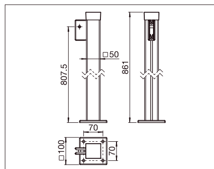
SR415/1 Kit poste para atornillar
