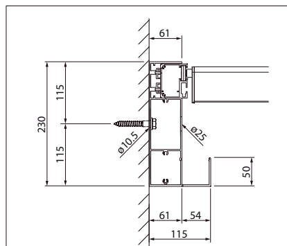
Sección perfil carril (wall mounting)
