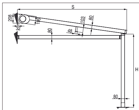
Sistema con portería
