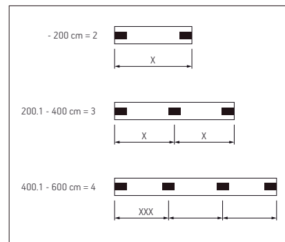
Reparto y nº de soportes (Cajón)
