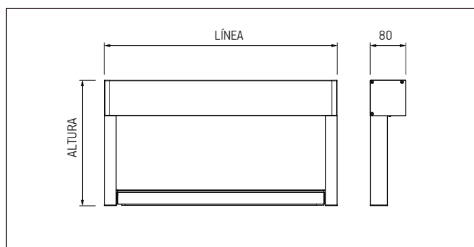
dimensiones máximas del sistema con guía
