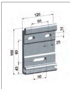
placa frontal - techo
