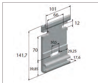
detalle soportes a muro
