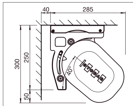
Instalación a techo 40°
