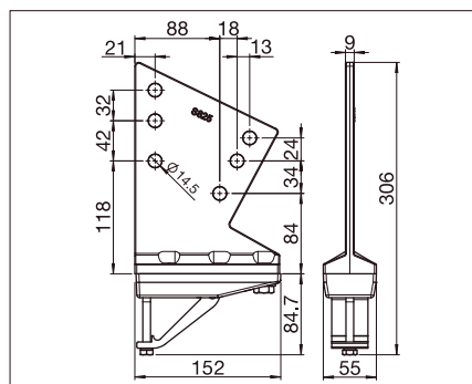
S825 Soporte para viga
