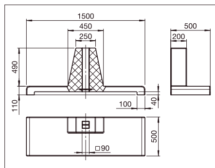
OS617 Zócalo de hormigón (ca. 186 kg)
