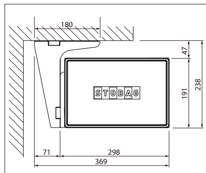
Montaje a techo
