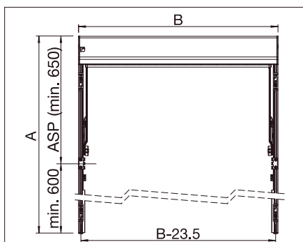
Plano de instalación W = anchura / ASP = Punto al descubierto
