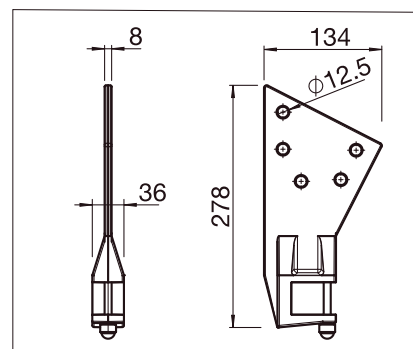
S225 Soporte de viga
