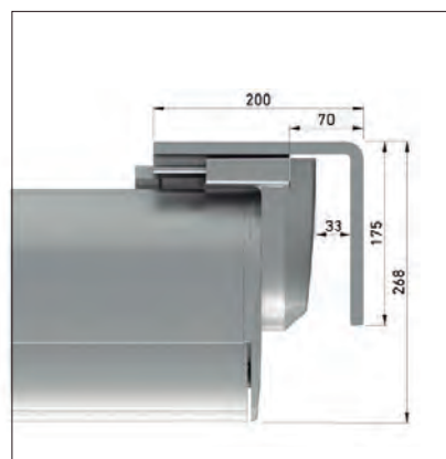
detalle sujeción entre paredes
