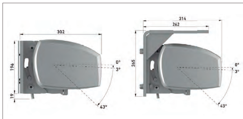
fijación a muro
