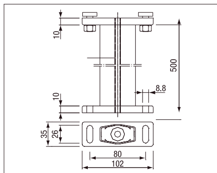
PS547 Soporte
