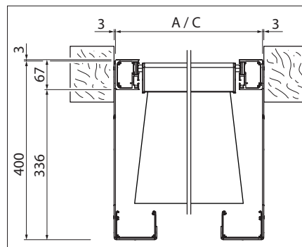
GP534 canalón opcional
