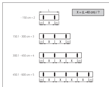
Reparto y nº de soportes sin ZIP
