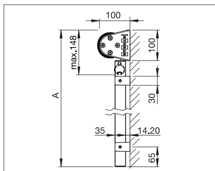
S4110/3 Montaje al frente
