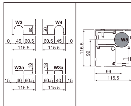
Detalle de drenajes
