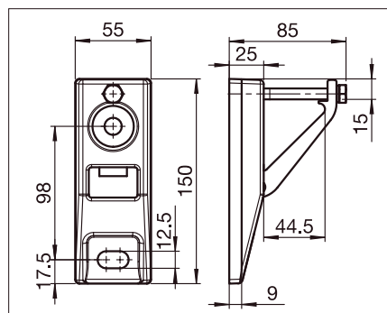
S821/2 Muro/soporte pequeño a techo
