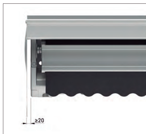
distancia recomendada entre tapas y soporte.
