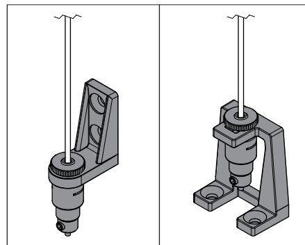
soporte de fijación a muro / suelo con tensor
