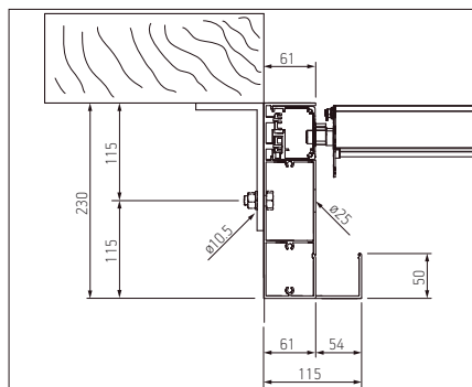
Sección del perfil del carril (a techo)
