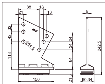
S725 Soportes para vigas
