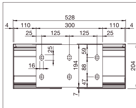
B423/2 Soporte de la guarnición 300 mm
