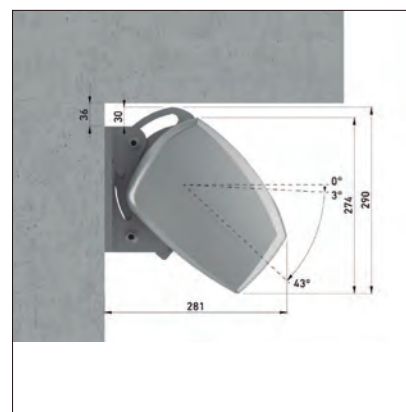
detalle espacio necesario para instalación
