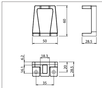
US120-1 Soporte de fijación a suelo
