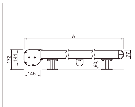
Instalación sobre estructura A = Proyección
