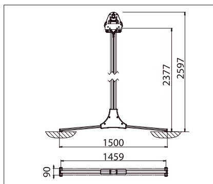
Version con 2 postes OS416/1 y pata transversal OS412
