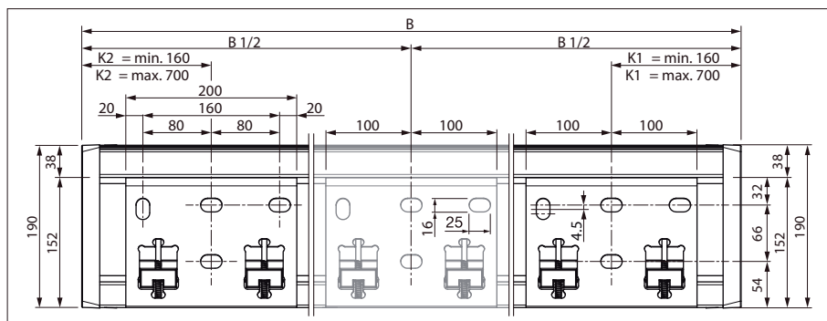
Plano de montaje (montaje a muro)
