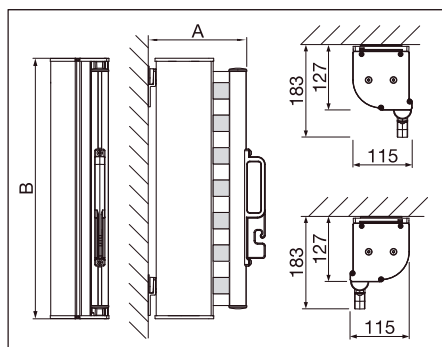
SR6000 Muro / Instalación superior
