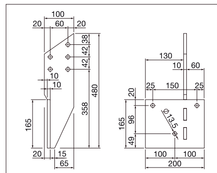
BX427 Soporte para vigas
