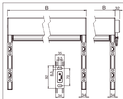
Disposición de los soportes, con soportes B = Total width
