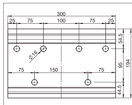
S563/2 Perfil de soporte L = 300
