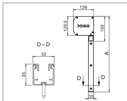
VS5200/2: Instalación a pared A = Altura total
