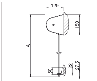
US3910/2 Instalación a pared
