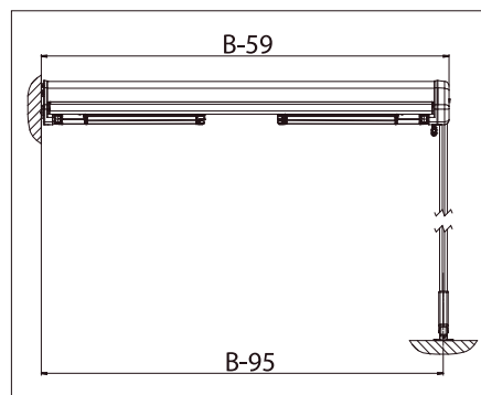
Version OS416/1 base de ángulo recto y transversal OS4010/1
