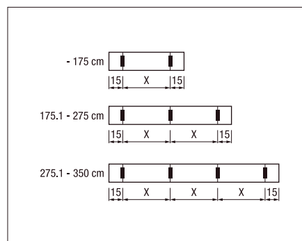
Posicionamiento y cantidad de soportes
