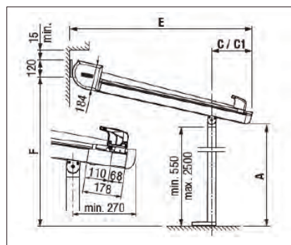
Montaje a muro con placa base
