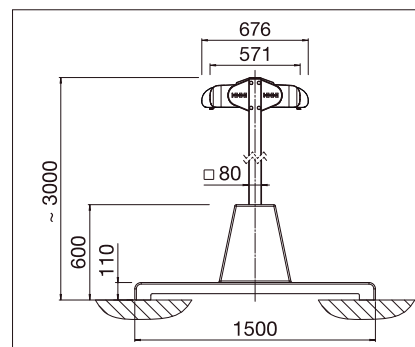
Vista lateral con estor de caída
