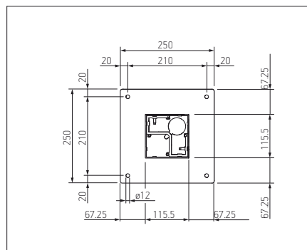
Placa base estándar
