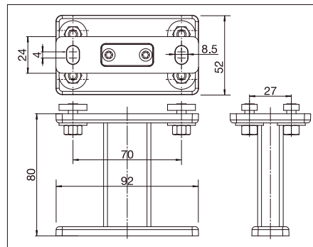
FS601/4 Soporte de fijación
