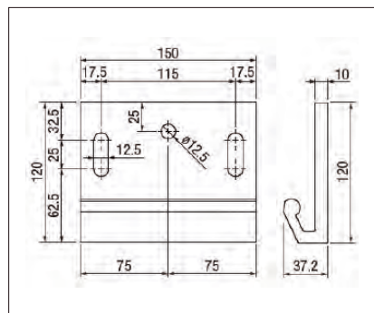
Soporte estándar
