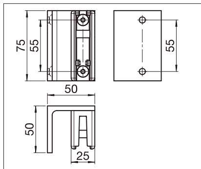
SR418 Conjunto de bisagras
