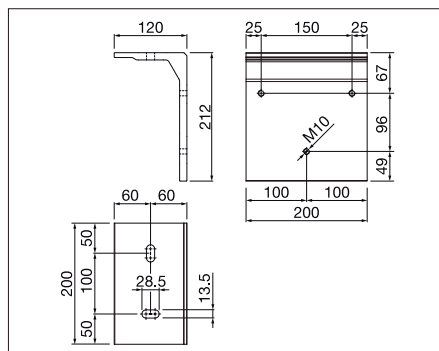
BX426 Herraje para montaje a techo
