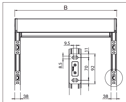
Plano de montaje: Montaje en pared con soportes de montaje B = Anchura total
