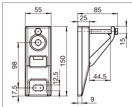
S821/2 Soportes pequeños techo/muro
