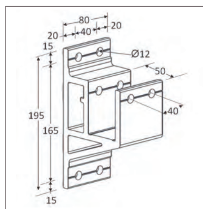
detalle soporte (frontal y a techo)
