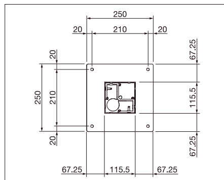
Sección placa suelo TP313 (Standard)
