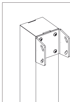
soporte exterior para guía y perfil 100x100
