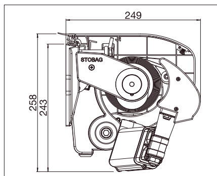
S8130/2 Instalación a pared con tejadillo S877/2
