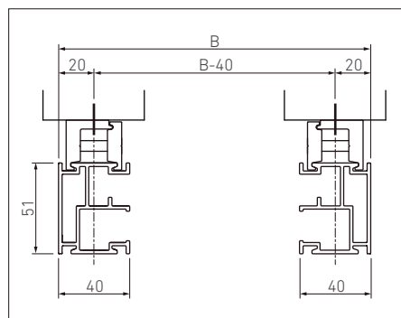
Vista de sección
