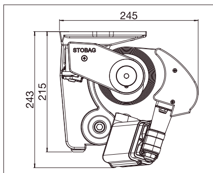
Instalación entre paredes
