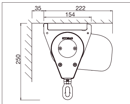
Instalación a techo Rail frontal redondeado
