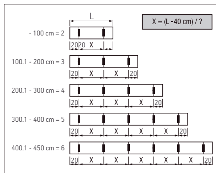
Reparto y nº de soportes (Rail guía)
