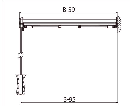
Version OS416/2 con taco a suelo y fijación a muro OS4010/1
