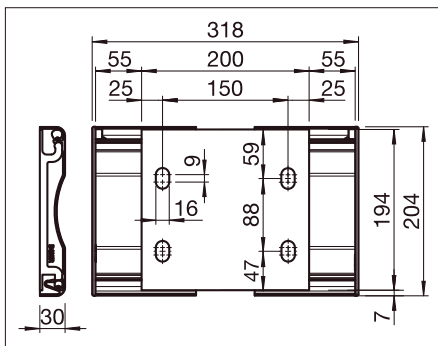
B423/1 Soporte de la guarnición 200 mm
