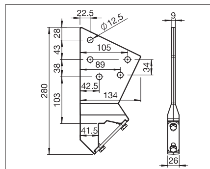
S825/1 Soportes para viga(vista frontal)
