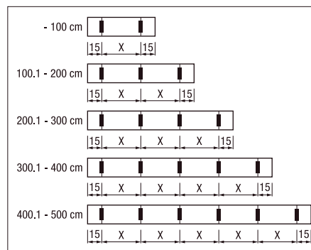
Disposición y número de soportes de montaje / punzones o clips
