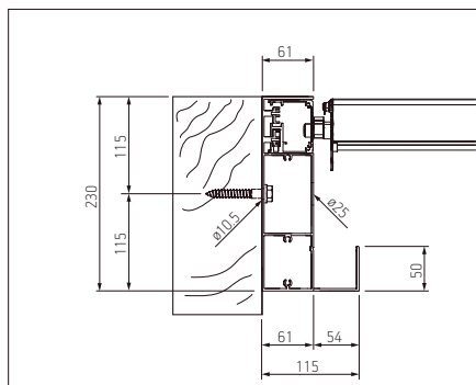
Sección del perfil del carril (entre paredes)
