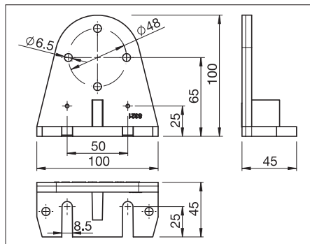
S321 Soporte combinado
