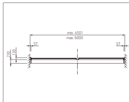
Vista frontal 2 módulos de techo TR4520
