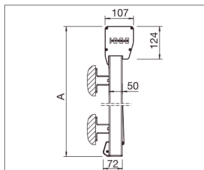
Al aire con cofre cuadrado
