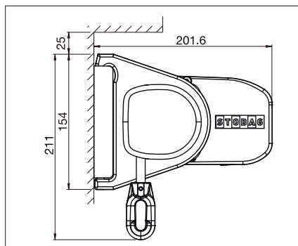
Instalación a pared Instalación con soportes S721/1
