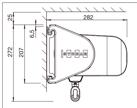
Vista lateral instalación a pared - redondeado
