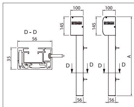
Montaje en fachada con soportes A = Altura total
