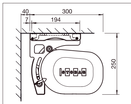
Instalación a techo
