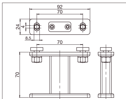
PS401/1 Soporte
