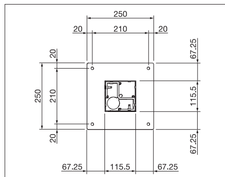
Sección de placa base TP313 (estándar)
