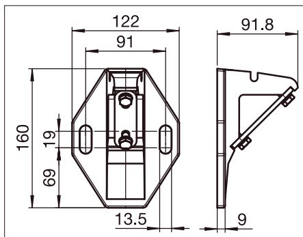
S831/3 Muro/ Soportes para techo(frontal)
