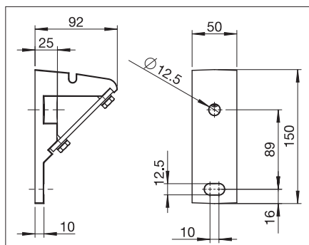
S831/5 Muro/Soportes pequeños para techo
