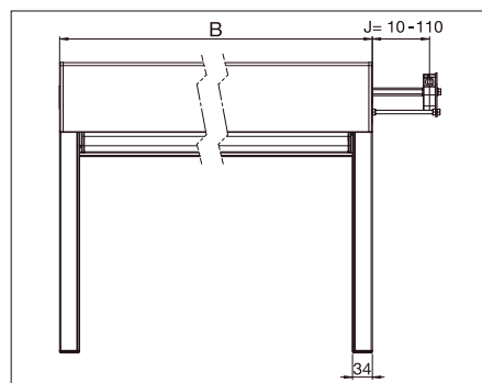
Disposición del soporte con el engranaje B = Total width
