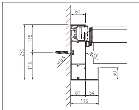
Sección del perfil del carril (entre paredes)
