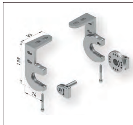
Detalle soportes
