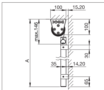
S4110/3 Montaje bajo techo
