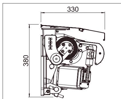
Instalación a pared con tejadillo opcional S247/3
