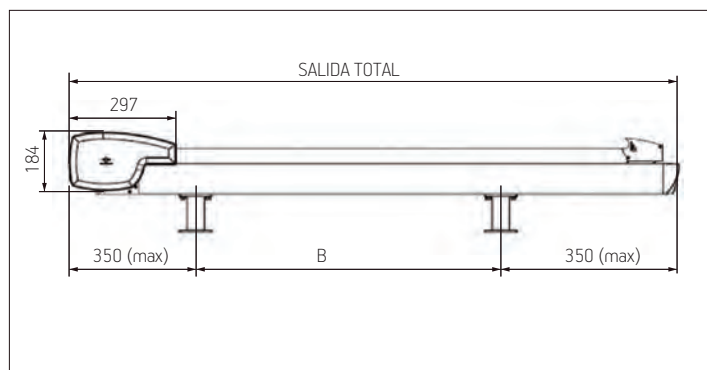
esquema de producto
