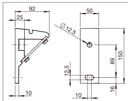
S831/5 Muro/ Soporte pequeño para techo(frontal)
