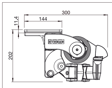
Instalación a techo sin tejadillo (S818 front rail)
