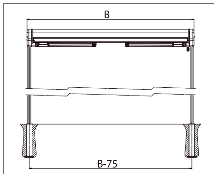
Version OS416/2 con taco a suelo OS315
