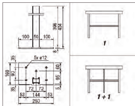
Placa base
