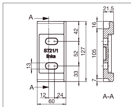
S721/1 Soporte
