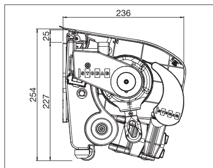
S8135 Instalación a muro
