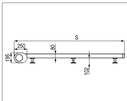
Vista lateral de producto
