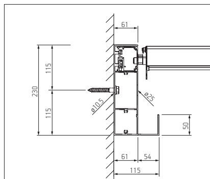
Sección perfil de soporte ( montaje a fachada)
