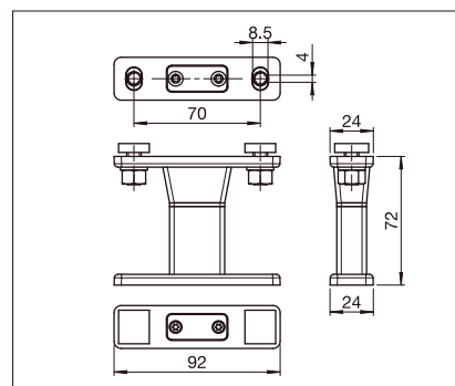
PS401/8 Soporte de fijación con Silent Block
