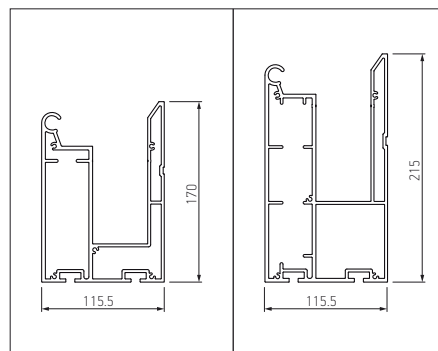
Modelos de canalón
