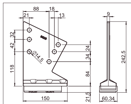
S725 Soporte para viga
