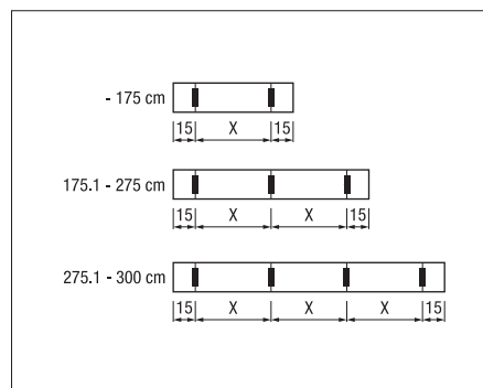
Reparto de soportes y puntos de fijación
