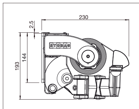
Instalación a pared sin tejadillo (S818 front rail)
