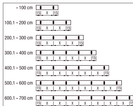
Configuración y número de abrazaderas de fijación
