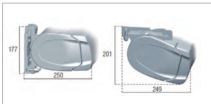
Motor y máquina - instalación a muro
