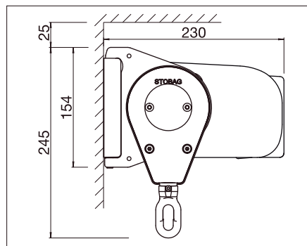
Instalación a pared Con rail frontal cuadrado
