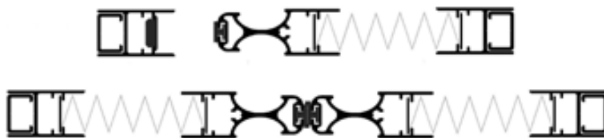
Detalle 2 hojas
